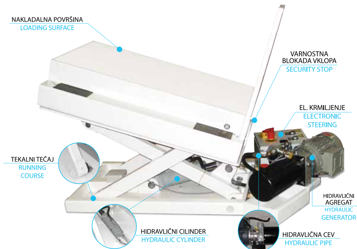
Hidravlična dvižna miza z naklonom / Hydraulic lifting table with gradient
