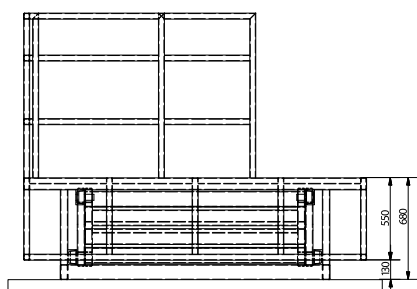
IZHODIŠČNI POLOŽAJ DVIŽNE PLOŠČADI STARTING POSITION
